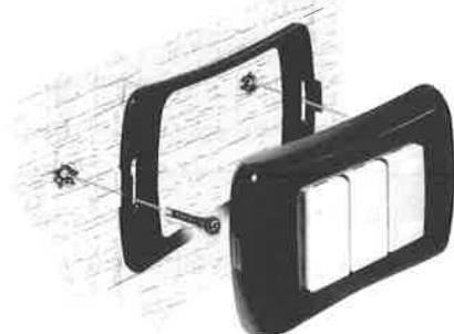
INSTALLAZIONE CON VITI SU PARETI RUSTICHE Utilizzare l'apposito supporto di fissaggio.
